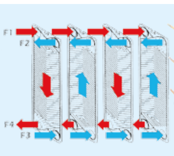
Circulation latérale à contre-courant
