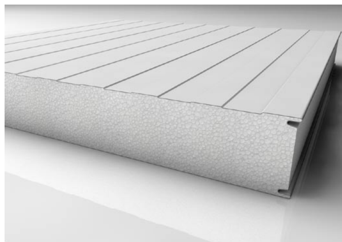
Panneaux faces nervurées
