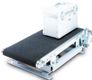
Balance, intégrée au convoyeur d'enregistrement
