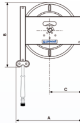
Flexible de raccordement de la machine eau chaude à l'enrouleur HP en option (DMG KITHP).
